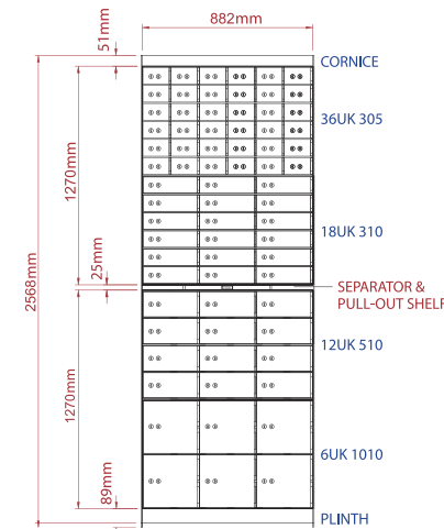
10 INCH MODULE
